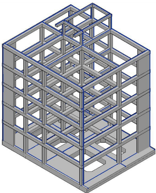
شکل ۸-۵-۱ اجرای شبکه همبندی اصلی در سقف خرپشته
