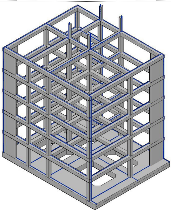
شکل ۷-۵-۱ اجرای شبکه همبندی اصلی در ستون‌های خرپشته
