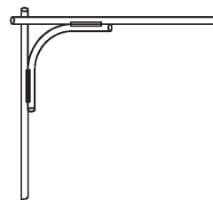
نحوه جوشکاری میلگردها در یک گوشه
