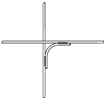
نحوه جوشکاری میلگردها در یک تقاطع چهارراهه
