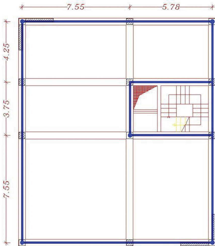
پلان همبندی تیپ طبقات
